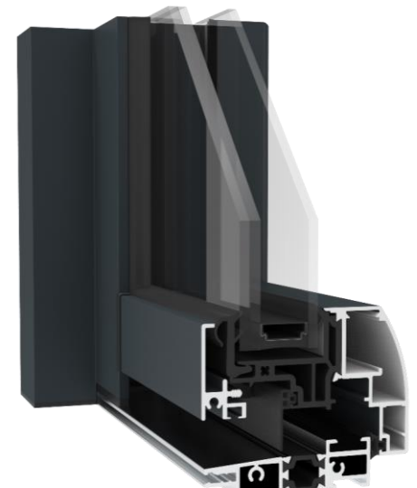
Seuil plat pour accès PMR
