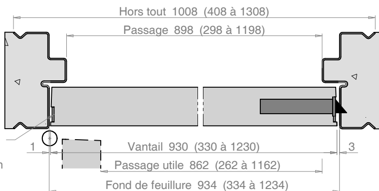
Ferrage représenté Universel 130x86 DU32
