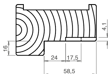
HUISSERIE FEUILLURE 58,5
