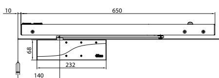
BCS2000.1 : Porte à 1 vantail
