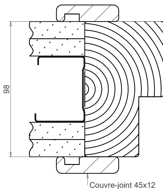
Huissérie représentée Feuilleure HU04 Section 98x57 sans rainure à brique
