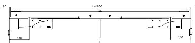
BCS2000.2 : Porte à 2 vantaux
