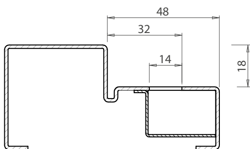
Coupe A-A
