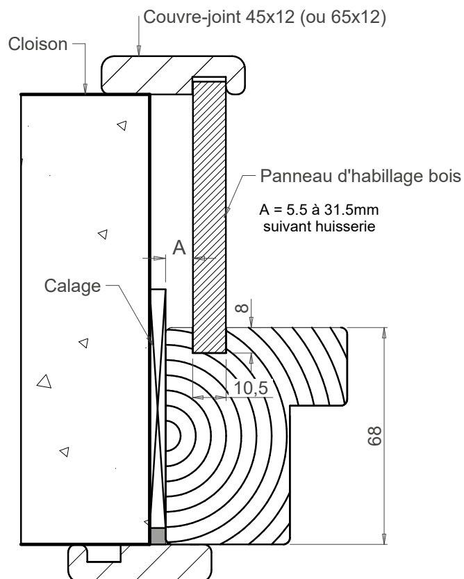
Huissérie Feuilleure HU04 Section 68x57 avec rainure d'ébrasement
